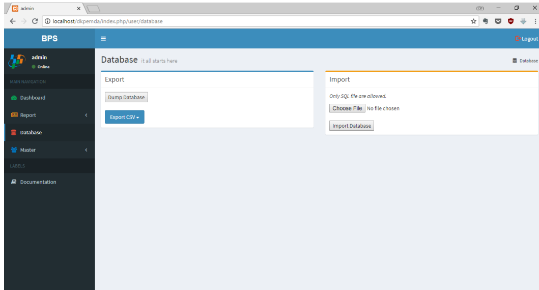
Gambar 27. Halaman database
