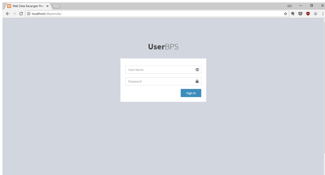
Gambar 18. Halaman login
